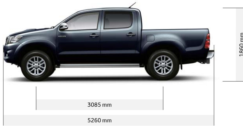
Abmessungen für Hilux 2,5 Doppelkabine City mit Radkastenverbreiterungen und 17" Leichtmetallfelgen.
